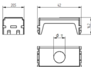
Saída de Fio
