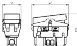
Interruptor Simples e Paralelo
